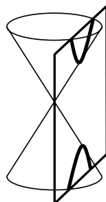
Hyperbel (besteht aus 2 Ästen)
