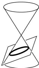
Ellipse (Sonderfall: Kreis)
