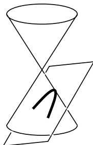
Parabel (Schnittebene parallel zur Seitenlinie)
